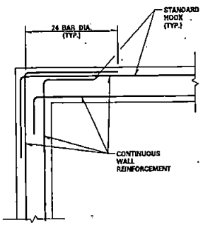
DETAIL A SCALE: 1" = 1'-0"
